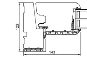
V20 Seitlicher Blendrahmen/Flügel
