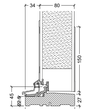
Einwärts öffnend, 45 mm Bodenschwelle, klar lackiertes Hartholz
