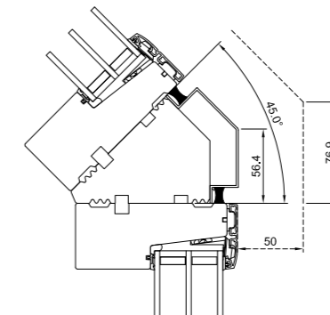
45° Eckpfosten
