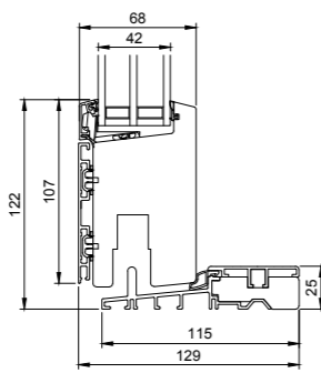
L34 Fußschwelle beweglicher Teil
