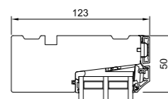
L6 Oberer Blendrahmen Oberlicht
