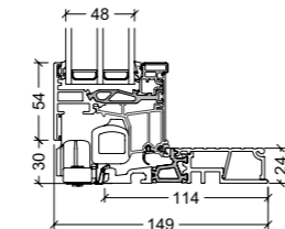
24 mm Alu/PA-Unterrahmen mit Alu-Trittschwelle, Schiebetür
