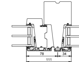
V11 Seitlicher Blendrahmen/ Seitenteil
