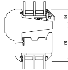
L8 Kämpfer; Flügel/ Oberlicht
