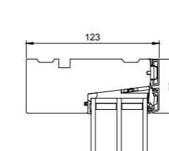
L6 Oberer Blendrahmen Oberlicht
