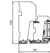
V1 Seitlicher Blendrahmen/ Flügel
