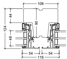
90 mm Pfosten (nur für Fenster)
