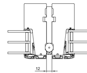
senkrecht mit 12 mm Fuge
