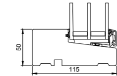
L28 Fußschwelle Seitenteil
