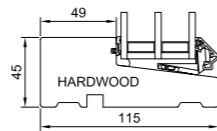
L28 Fußschwelle Seitenteil aus Holz
