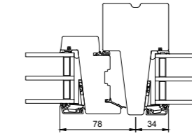
V11 Seitlicher Blendrahmen/Seitenteil
