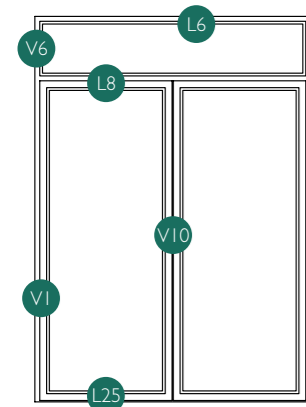
L6 Oberer Blendrahmen Oberlicht
