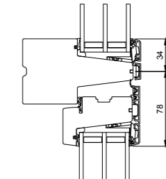
L8 Kämpfer; Flügel/ Oberlicht
