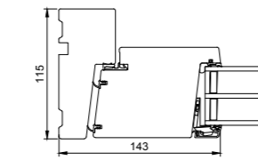
V20 Seitlicher Blendrahmen/Flügel
