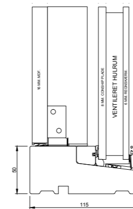
Ventilierte Füllung unterer Blendrahmen
