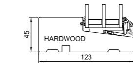
L25 Fußschwelle Seitenteil aus Holz
