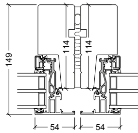
VELFAC 200 ENERGY - VELFAC 200 ENERGY Waagerechte Kopplung
