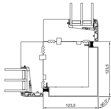
90° Eckpfosten
