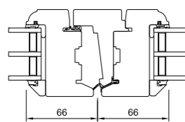
V10 Mittlerer Anschlag Stulp
