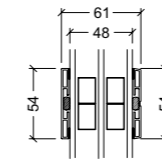
54 mm Energiesprosse 3-fach Verglasung
