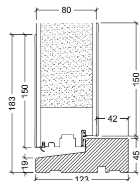
Auswärts öffnend, 45 mm Bodenschwelle, klar lackiertes Hartholz
