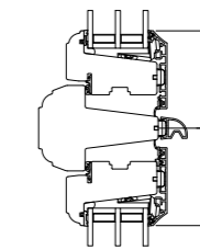
L10 Kämpferprofil
