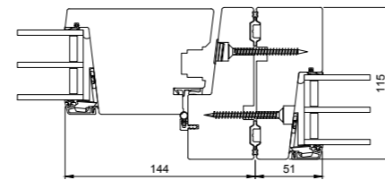
V26 Seitlicher Blendrahmen, Schließseite/Seitenteil
