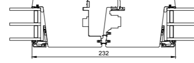
V22 Stulpausführung
