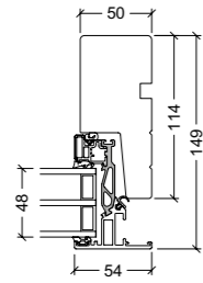
Seitenrahmen
