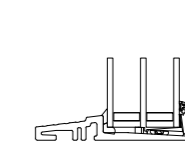
L28 Fußschwelle Seitenteil Standard
