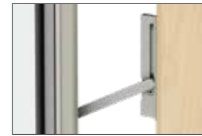
Öffnungsbegrenzer, abschließbar. Darf nicht in Rettungswegfunktion eingesetzt werden. Nicht für Schiebetüren erhältlich. In einer Länge von 160mm und 270mm erhältlich.
