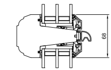
S2 Sprosse
