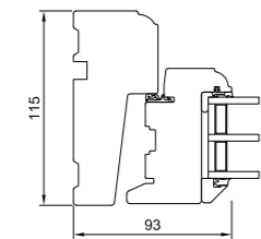
V1 Seitlicher Blendrahmen/ Flügel
