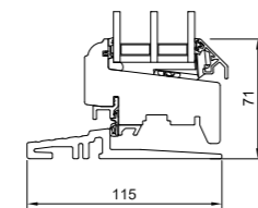
L25 Fußschwelle Standard
