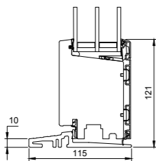
L25 Fußschwelle Standard
