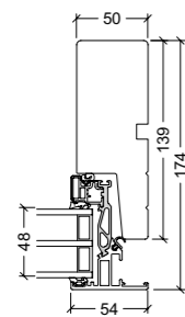
139 mm Rahmen
