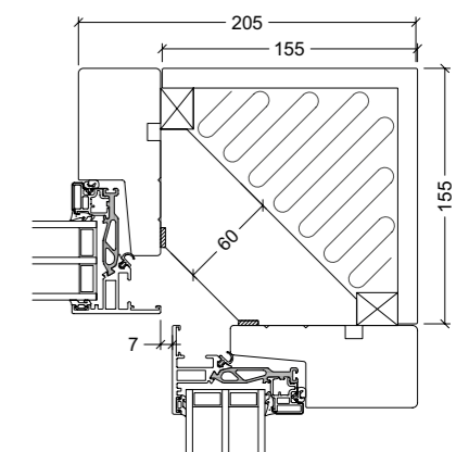
90° Innenecken Holz Typ A2014
