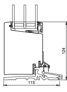
L25 Fußschwelle
