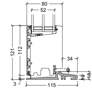
Auswärts öffnend, 18 mm Bodenschwelle, HELO®
