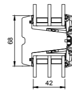
Sprosse
