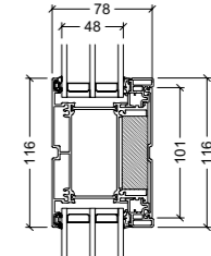
116 mm glasteilende Sprosse 3-fach Verglasung
