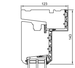
L20 Oberer Blendrahmen/Flügel
