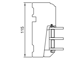
V6 Seitlicher Blendrahmen Oberlicht
