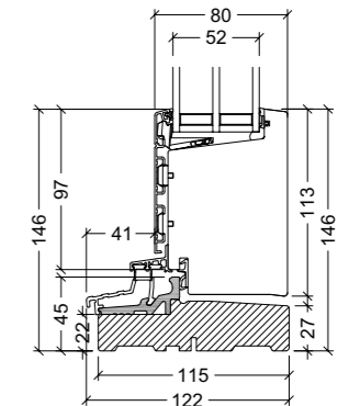
Einwärts öffnend, 45 mm Bodenschwelle, klar lackiertes Hartholz
