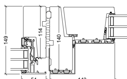
VELFAC 200 ENERGY - VELFAC Ribo Einwärts öffnende Tür
