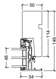
114 mm Rahmen
