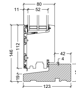
Auswärts öffnend, 45 mm Bodenschwelle, klar lackiertes Hartholz
