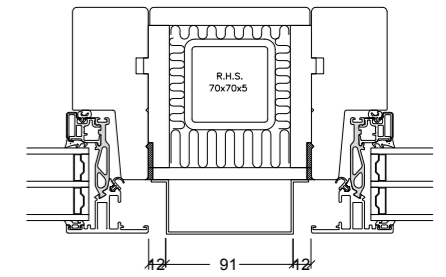
Beispiel auf Säulelösung Alu-Abdeckung Typ A3011
