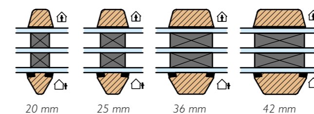
Softline Profil
