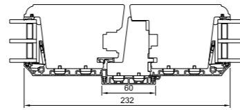
V22 Stulpausführung
