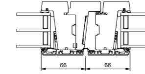
V10 Mittlerer Anschlag Stulp
