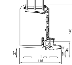
L25 Fußschwelle Holz
