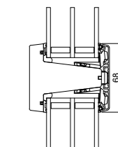
68 mm Sprosse
