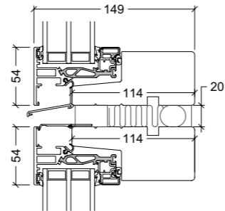
VELFAC 200 ENERGY - VELFAC 200 ENERGY Senkrechte Kopplung mit Wassernase. Bei Kopplungen von VELFAC Fenstern über mehrere Stockwerke ist eine Wassernase alle 3000-3500 mm erforderlich.
