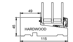
L28 Fußschwelle Seitenteil Holz
