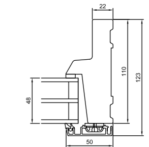
L6 Seitlicher Blendrahmen Unterlicht
