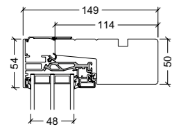
Oberrahmen
