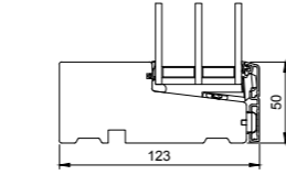
L28 Fußschwelle Seitenteil Holz
