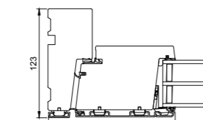
V20 Seitlicher Blendrahmen/ Flügel
