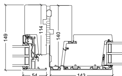
VELFAC 200 ENERGY - VELFAC Ribo Auswärts öffnende Tür
