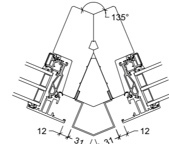
45° Außenecke Holz Typ A2202, Alu-Abdeckung Typ A1202
