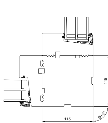
90° Eckpfosten
