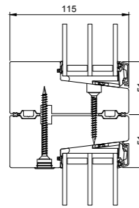
L7 Kämpferprofil
