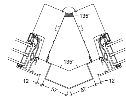
45° Außenecke Holz Typ A2201, Alu-Abdeckung Typ A1201
