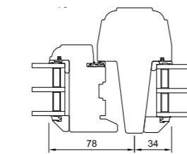
V3 Seitlicher Blendrahmen/ Seitenteil
