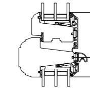
L11 Fester Blendrahmen/Flügel
