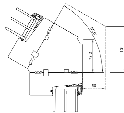
60° Eckpfosten
