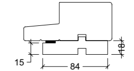
Auffütterung Typ 18-84
