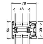
54 mm glasteilende Sprosse 3-fach Verglasung
