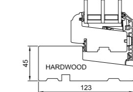
L25 Fußschwelle Holz
