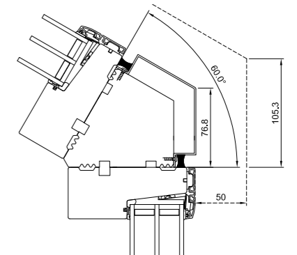
60° Eckpfosten
