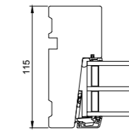
V6 Seitlicher Blendrahmen Oberlicht
