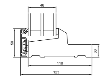
L3 Fußschwelle Unterlicht
