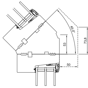
45° Eckpfosten
