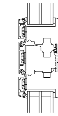
V22 Stulpausführung
