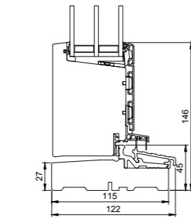
L25 Fußschwelle Tür Holz
