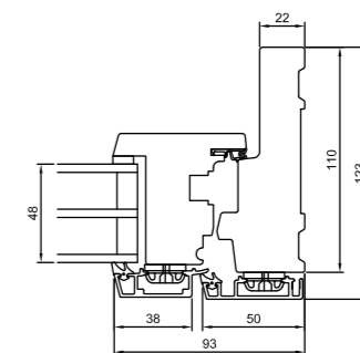
V1 Seitlicher Blendrahmen/Flügel
