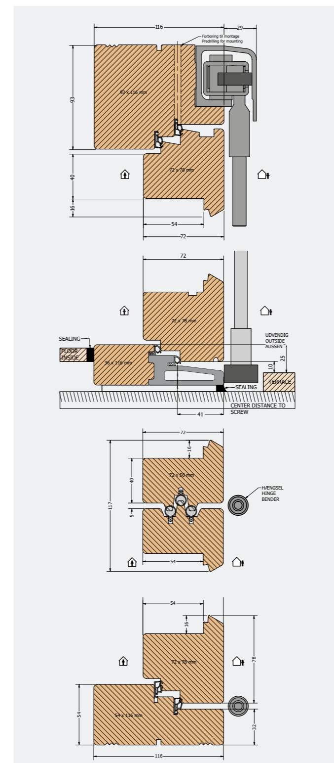
Softline Profil
