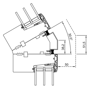
30° Eckpfosten
