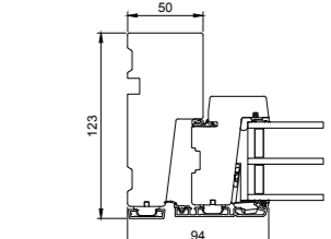
V1 Seitlicher Blendrahmen/ Flügel
