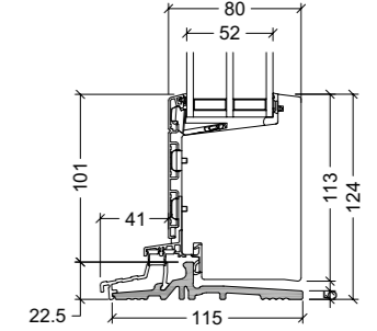
Einwärts öffnend, 22,5 mm Bodenschwelle, HELO®
