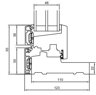
L25 Fußschwelle Holz
