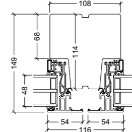
114 mm Pfosten (Kämpfer)
