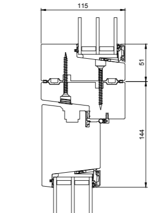
L27 Oberer Blendrahmen, Flügel/Oberlicht
