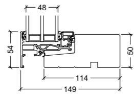
Unterrahmen
