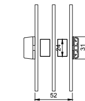
31 mm Sprosse
