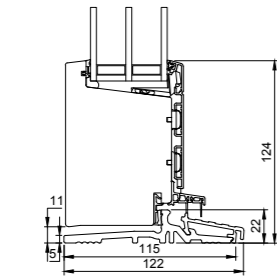
L25 Fußschwelle Tür Standard
