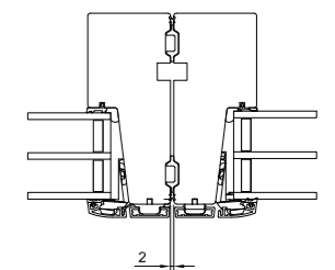
senkrecht mit 2 mm Fuge
