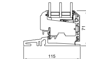
L25 Fußschwelle Standard
