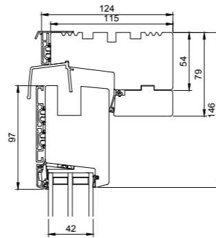
L32 Oberer Blendrahmen mit Flügel
