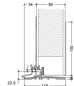
Einwärts öffnend, 22,5 mm Bodenschwelle, HELO®
