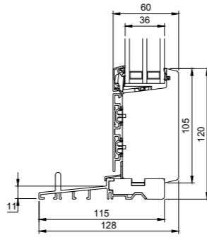
L33 Fußschwelle fester Teil
