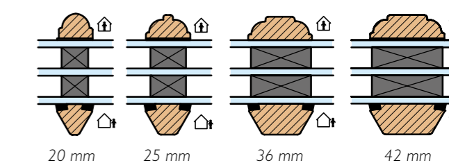
Bauernhausprofil
