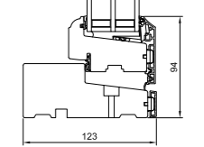
L9 Unterer Blendrahmen/ Flügel
