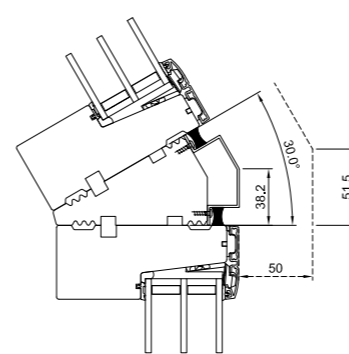
30° Eckpfosten
