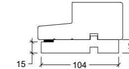
Auffütterung Typ 18-104
