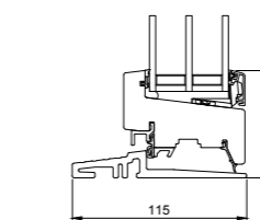
L25 Fußschwelle Tür Standard
