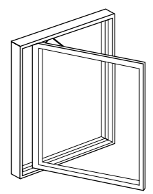
Flügel dreht sich bis zu 80° nach außen und ermöglicht das Putzen von innen
