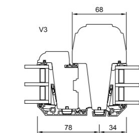
V3 Seitlicher Blendrahmen/Seitenteil
