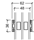
36 mm Energiesprosse 3-fach Verglasung
