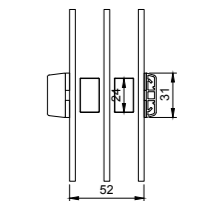
31 mm Sprosse
