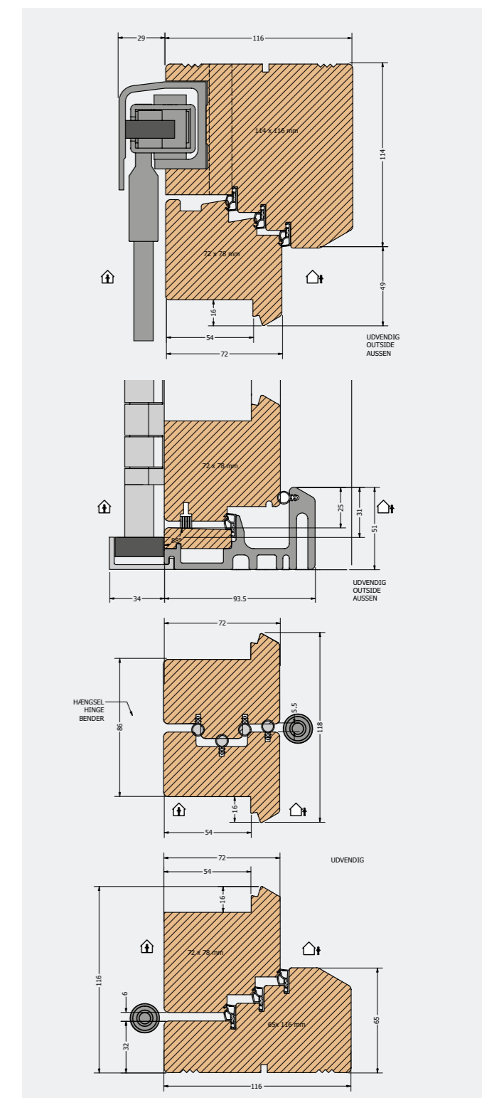
Bauernhausprofil
