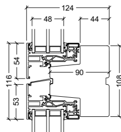
90 mm Kämpfer
