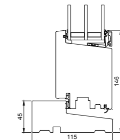
L25 Fußschwelle Holz
