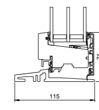
L25 Fußschwelle Tür Standard
