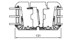
V10 Mittlerer Anschlag Stulp
