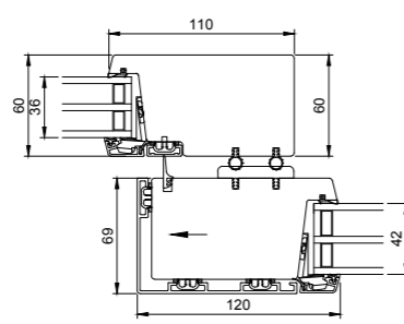
V31 Mittelposten/Flügel
