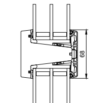
68 mm Sprosse
