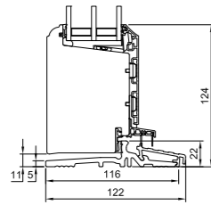
L25 Fußschwelle Standard
