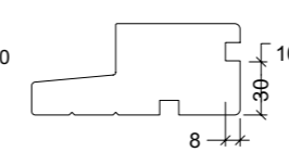
Nut typ 30-10-8
