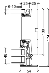
139 mm Rahmen mit Vorsatzflügel
