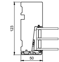
V6 Seitlicher Blendrahmen Oberlicht
