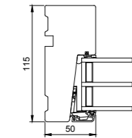
V6 Seitlicher Blendrahmen
