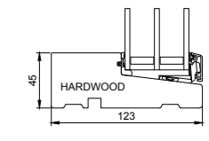
L28 Fußschwelle Seitenteil Holz
