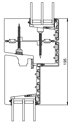
L27 Oberer Blendrahmen, Flügel/Oberlicht
