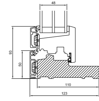
L25 Fußschwelle Hartholz
