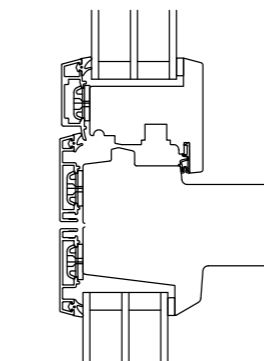
L9 Kämpferprofil Flügel/Festelement
