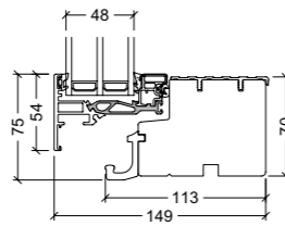
70 mm Unterrahmen mit Alu-Trittschwelle, Schiebetür
