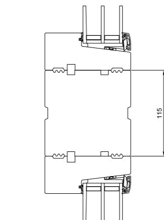
180° Pfosten
