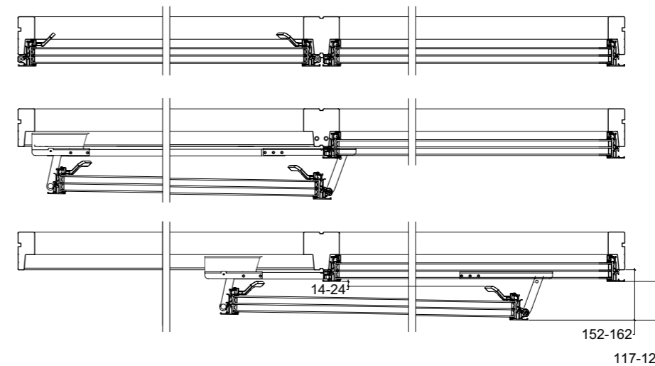
Öffnungsfunktion der Schiebetür mit 25 mm Bodenschwelle
