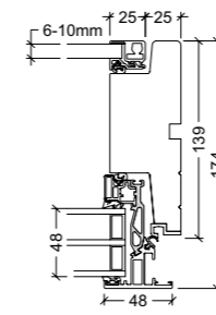
139 mm Rahmen mit Vorsatzflügel für Wendefenster ohne Überschlag
