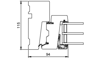
V1 Seitlicher Blendrahmen/Flügel
