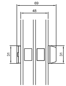
31 mm Sprosse
