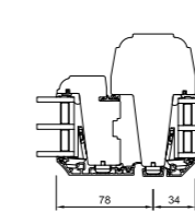
V4 Fester Blendrahmen/Flügel
