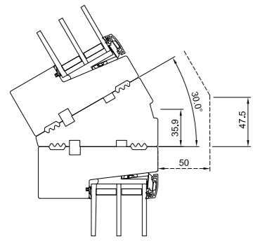
30° Eckpfosten
