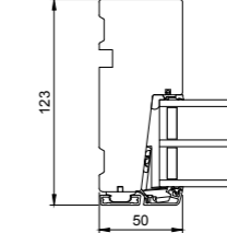
V6 Seitlicher Blendrahmen Oberlicht
