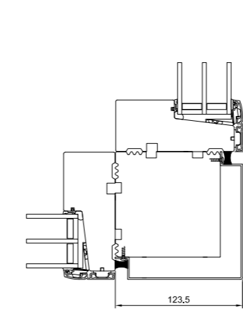
90° Eckpfosten
