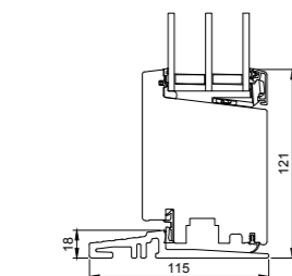
L25 Fußschwelle Standard
