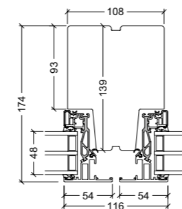
139 mm Pfosten (Kämpfer)
