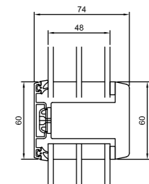
60 mm Sprosse
