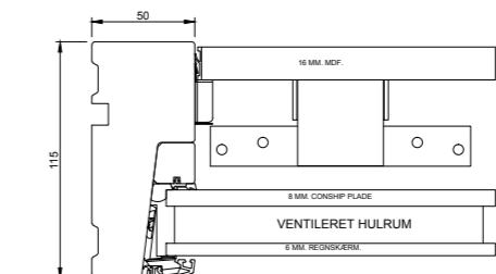
Ventilierte Füllung seitlicher Blendrahmen
