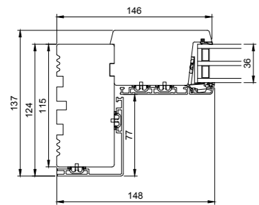
V30 Seitlicher Blendrahmen fester Teil
